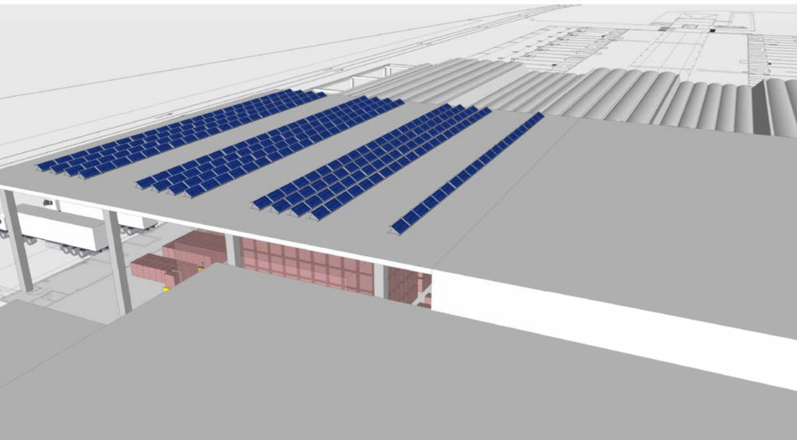
TIPOLOGICO IMPIANTO FOTOVOLTAICO
