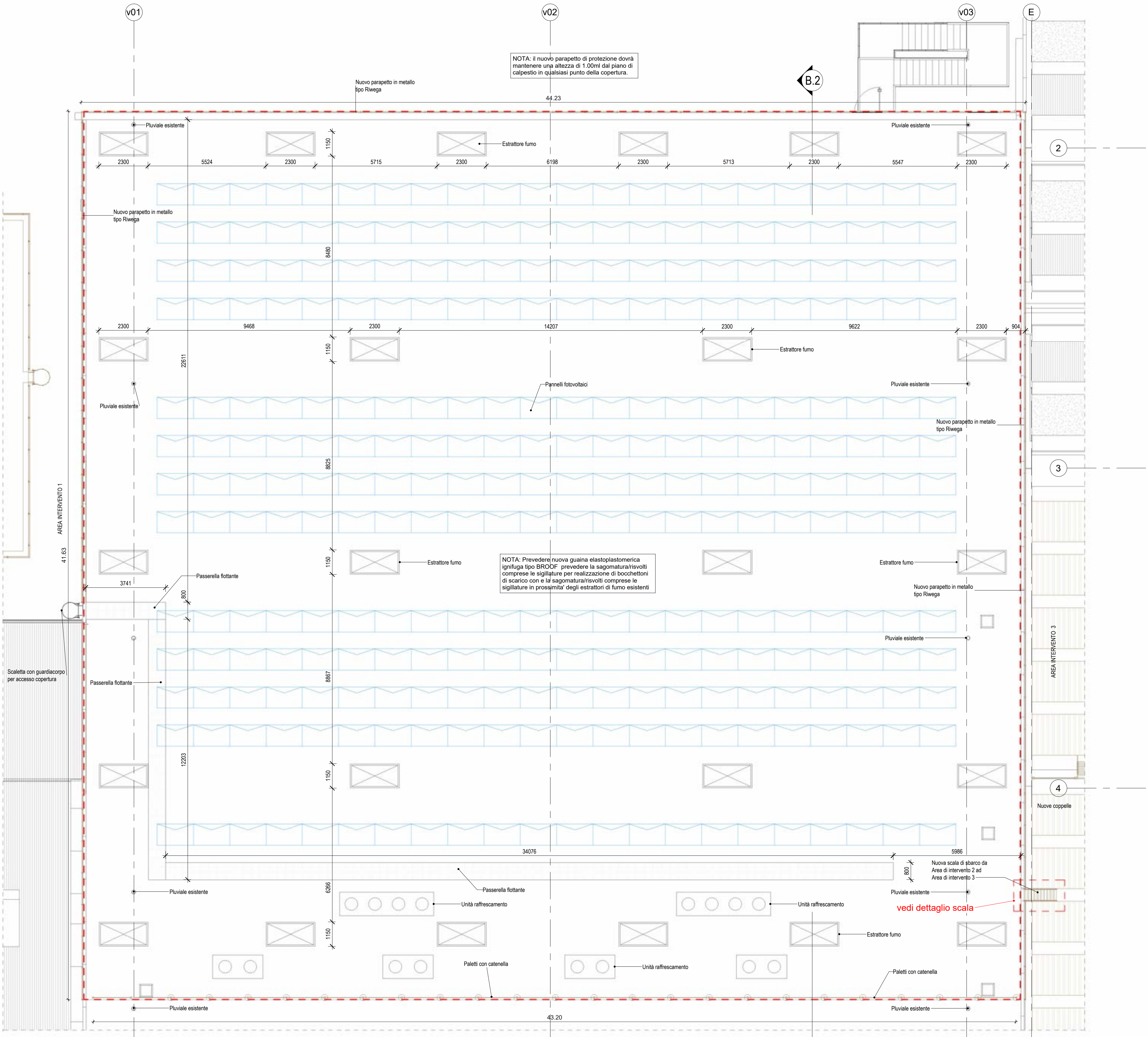
PIANTA DELLA COPERTURA
