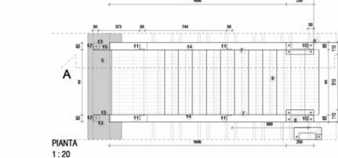
SCALA SBARCO COPERTURA INT.2:INT.3
